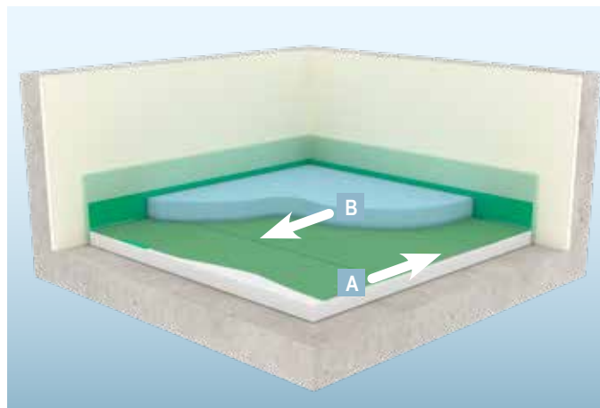
Grafika 27: Kierunek układania warstwy papieru parafinowego Knauf i kierunku wylewania płynnego podkładu anhydrytowego
