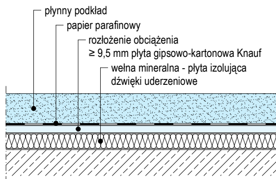
F231.pl-V104 Płynny podkład na izolacji z wełny mineralnej
