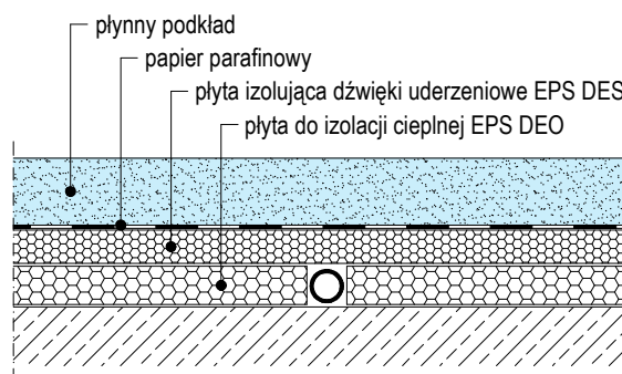
F231.pl-V106 Zmiana wysokości podkładu
