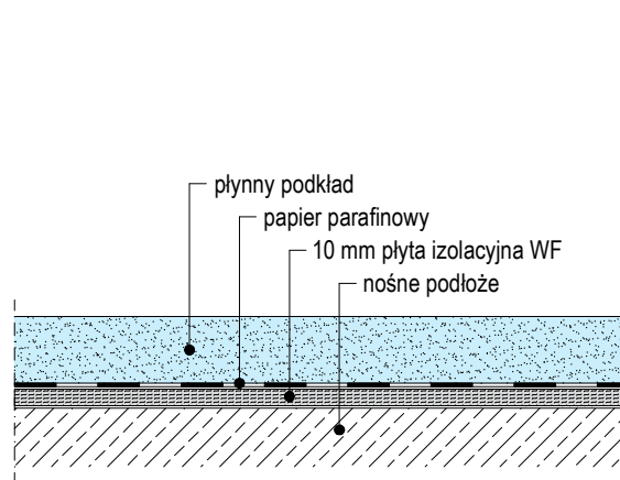
F231.pl-V114 Wyrównanie podłoża za pomocą podsypki
