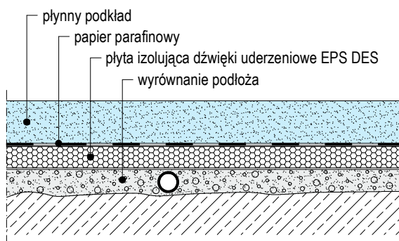
F231.pl-V105 Płynny podkład na izolacji termicznej lub od dźwięków uderzeniowych
