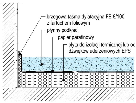
F231.pl-V105 Płynny podkład na izolacji termicznej lub od dźwięków uderzeniowych
