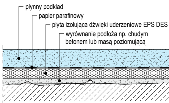
F231.pl-V103 Wyrównanie podłoża chudym betonem lub masą poziomującą
