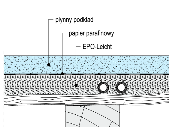
F231.pl-V115 Wyrównanie podłoża za pomocą EPO-Leicht
