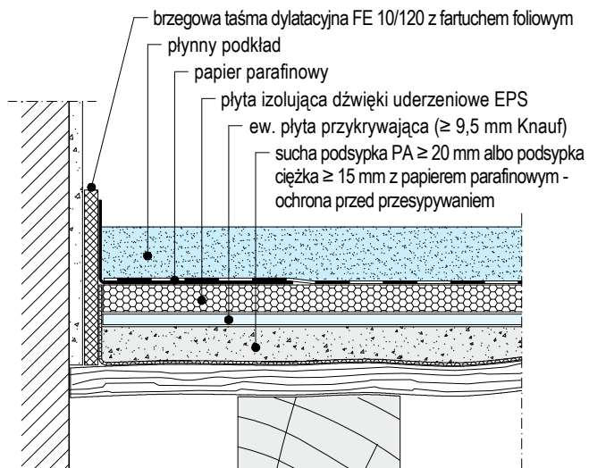
F231.pl-V109 Płynny podkład na izolacji termicznej / od dźwięków uderzeniowych
